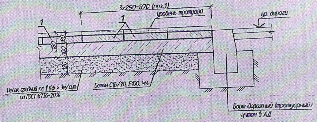
Лоток водоотводной тип 1 Разрез 2-2
