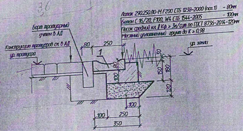
Лоток водоотводной тип 1 Разрез 1-1
